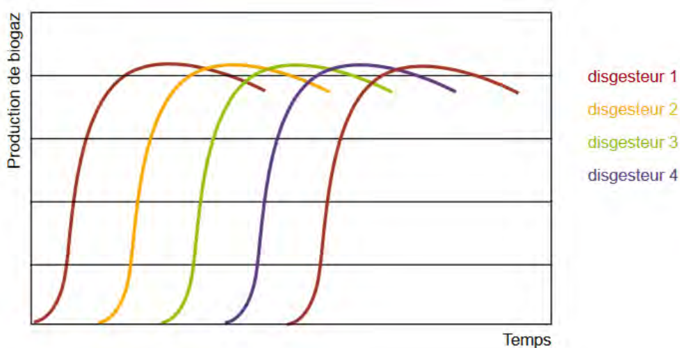
Figure 1 : Schéma représentatif de la production de biogaz dans le temps, pour un procédé voie sèche discontinu
