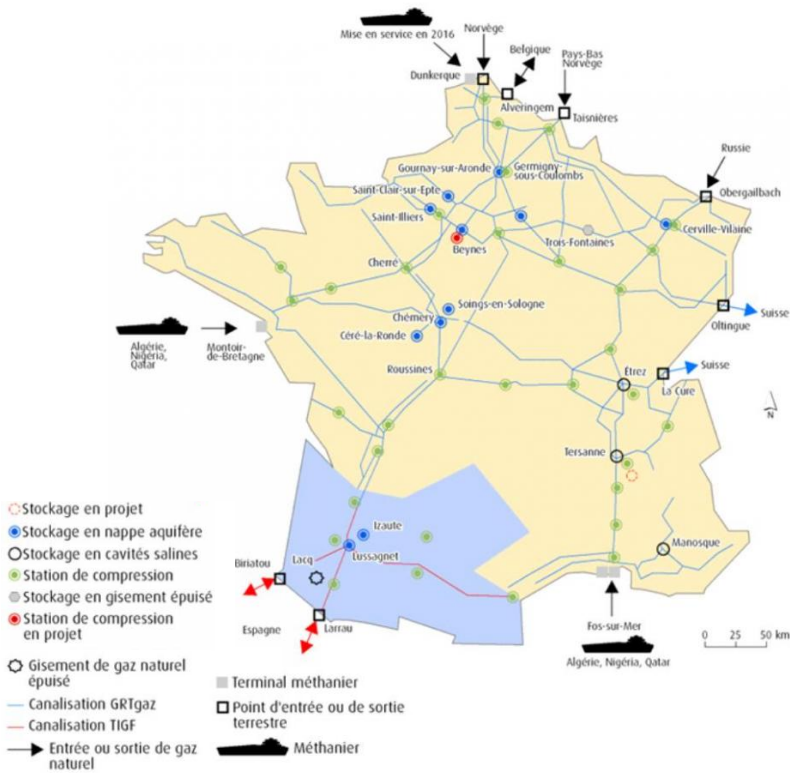
Figure 3 : points d'interconnexion et terminaux méthaniers
