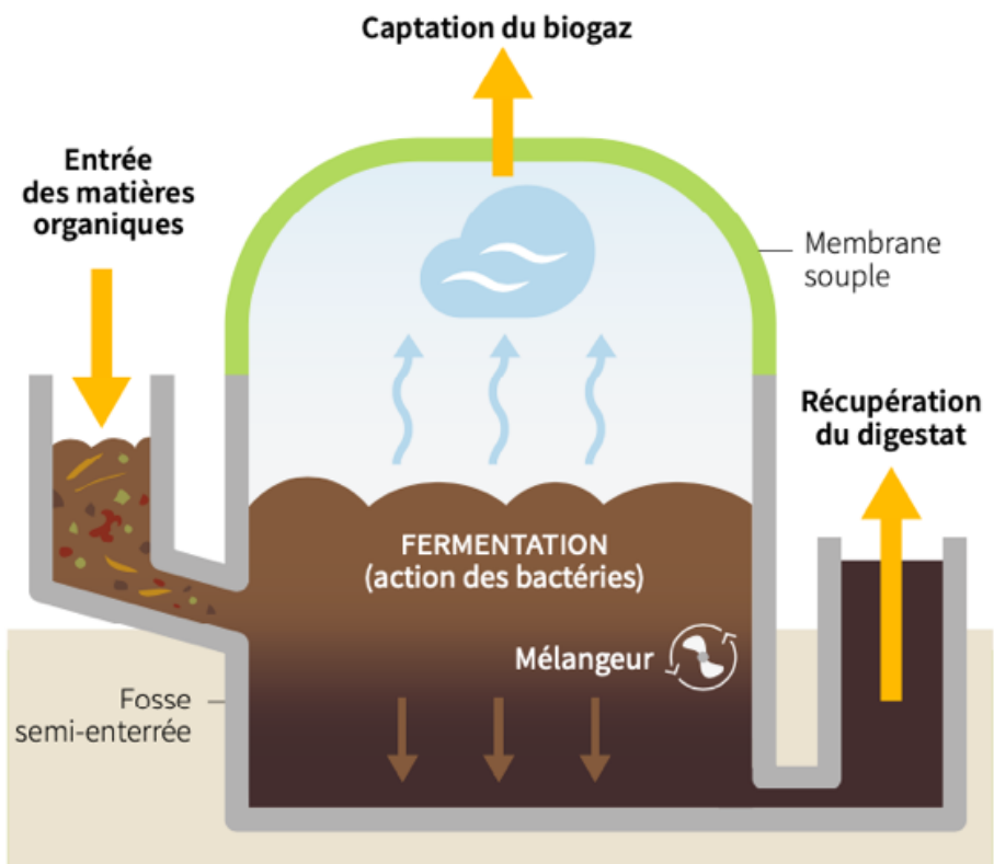
Figure 8 : Fonctionnement d'un méthaniseur (en anaérobiose à 38°)
